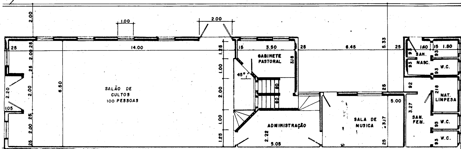
PLANTA
