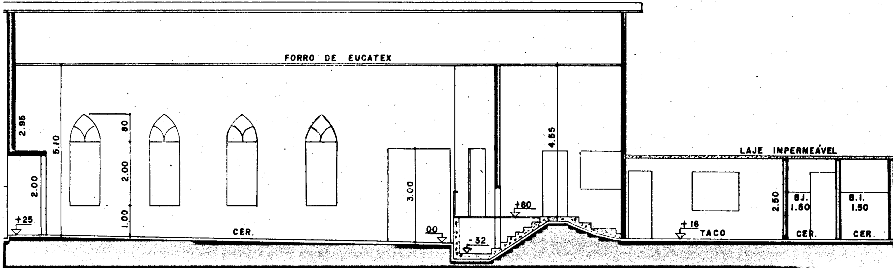
CORTE A-A
